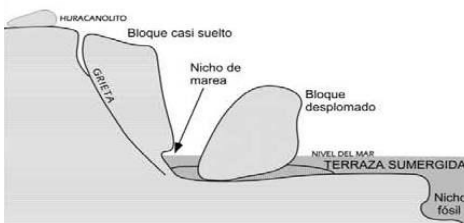
E-Esquema del proceso de desprendimiento de bloques desde los frentes de terraza. Estos bloques pueden ser lanzados tierra adentro por oleaje extremo.
